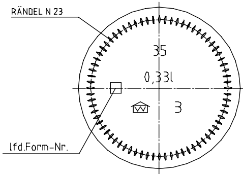
BODENANSICHT
